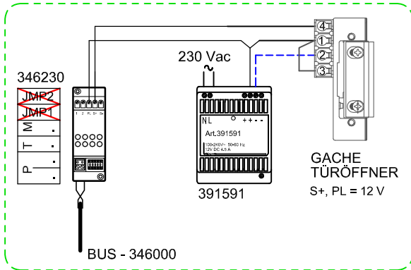
RELAIS 346230
