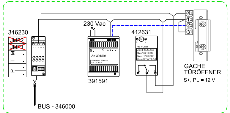
RELAIS 346230
