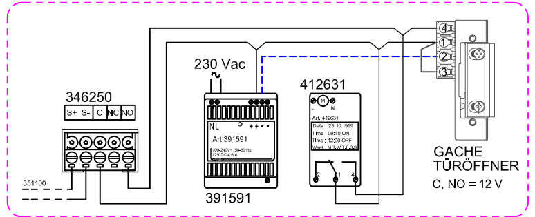
RELAIS 346250
