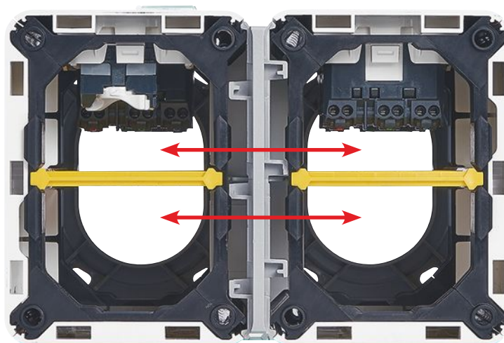
Ansicht von oben von zwei verbundenen Minisäulen
